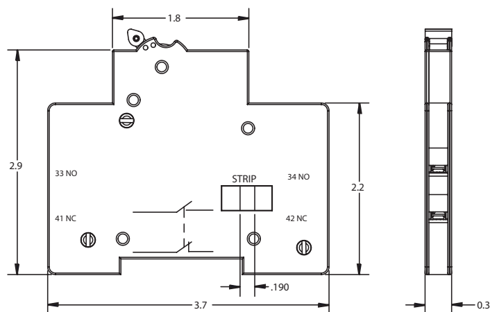
CCP2-AUX-100
