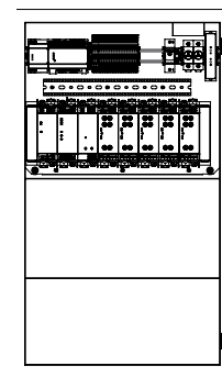
DualGuard-S4C3
