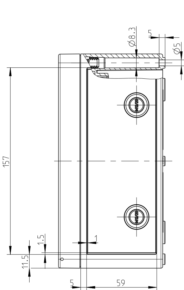
D-D
