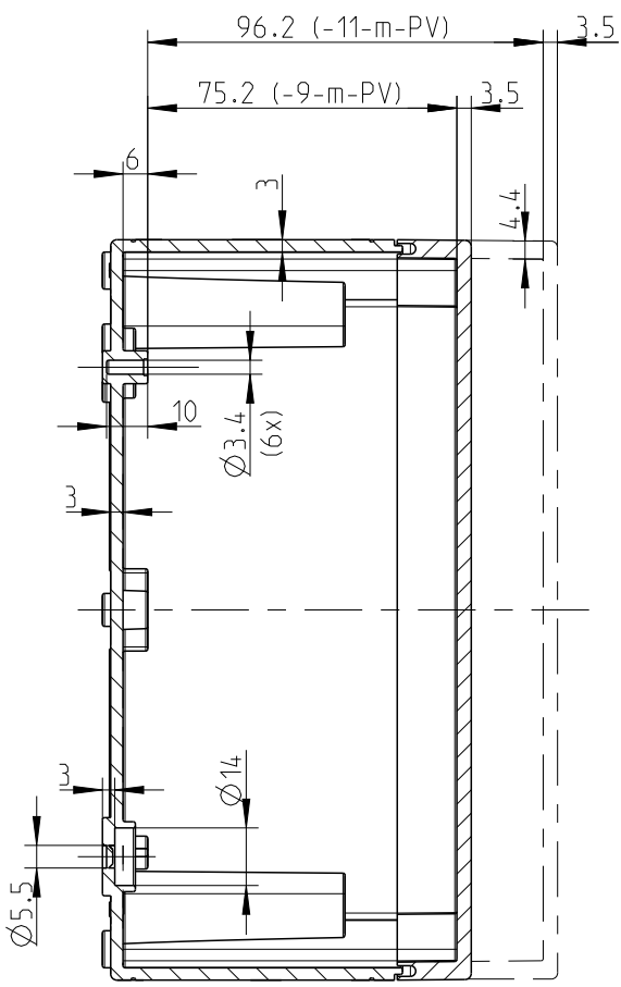
A-A
