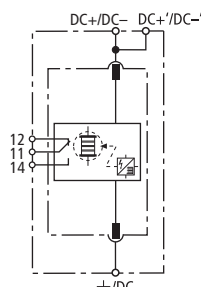
Schéma vnitřního zapojení
