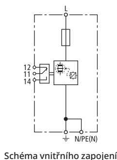
Schéma vnitřního zapojení
