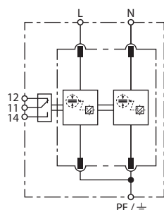
Schéma vnitřního zapojení
