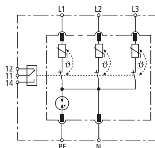
Schéma vnitřního zapojení
