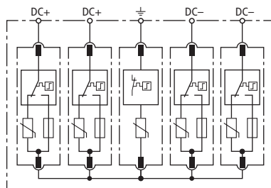
Schéma vnitřního zapojení
