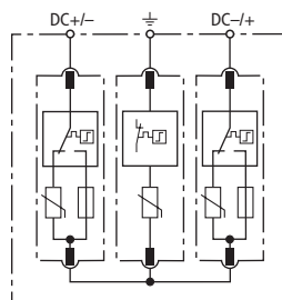
Schéma vnitřního zapojení
