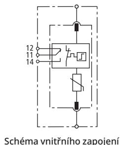
Schéma vnitřního zapojení
