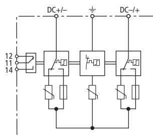
Schéma vnitřního zapojení
