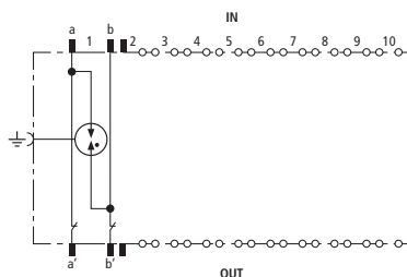
Schéma vnitřního zapojení
