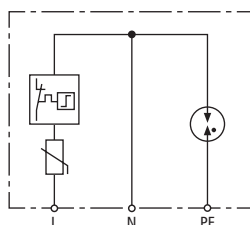
Schéma vnitřního zapojení
