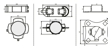
Rozměry
