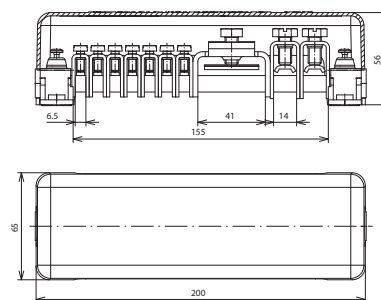
Rozměry
