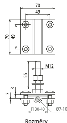
Rozměry
