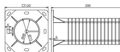
Rozměry
