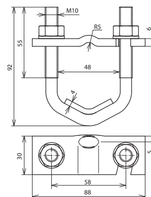
Rozměry
