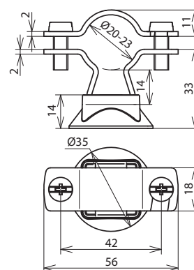
Rozměry
