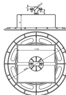
Rozměry
