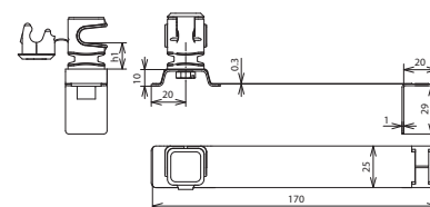
Rozměry
