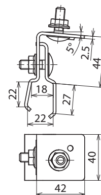
Rozměry
