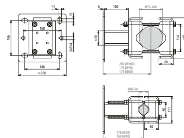
Rozměry
