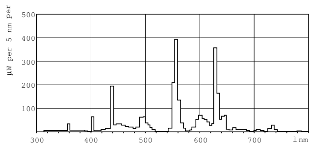
Barva světla /840
