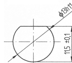
Tvar klíče
