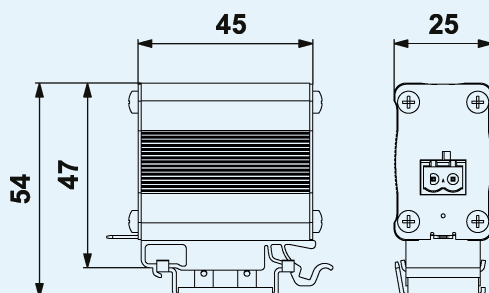
Rozměry produktu
