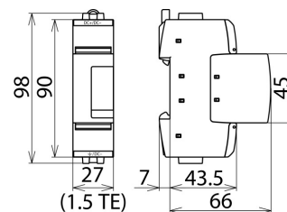
Rozměry DG SE DC 60
