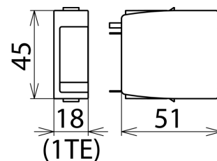
Rozměry DR MOD 255
