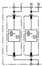
Schéma vnitřního zapojení DV M TN 255
