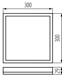
AZPO LED 17,5W
