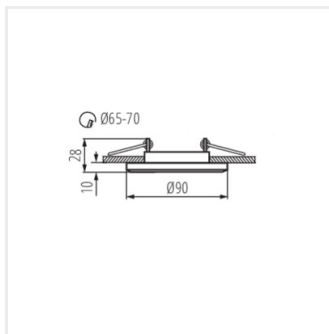
MORTA CT-DSO50
