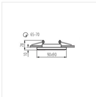
MORTA CT-DSL50
